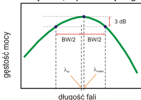
Rys. 5. Schematyczne pokazanie punktu mocy maksymalnej \lambda_{\text{maks}} oraz średniej długości fali \lambda_{\text{śr}} oraz szerokości pasma optycznego, BW — szerokość pasma optycznego
