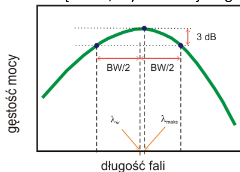
Rys. 5. Schematyczne pokazanie punktu mocy maksymalnej \lambda_{maks} oraz średniej długości fali średniej długości fali, BW — szerokość pasma optycznego
